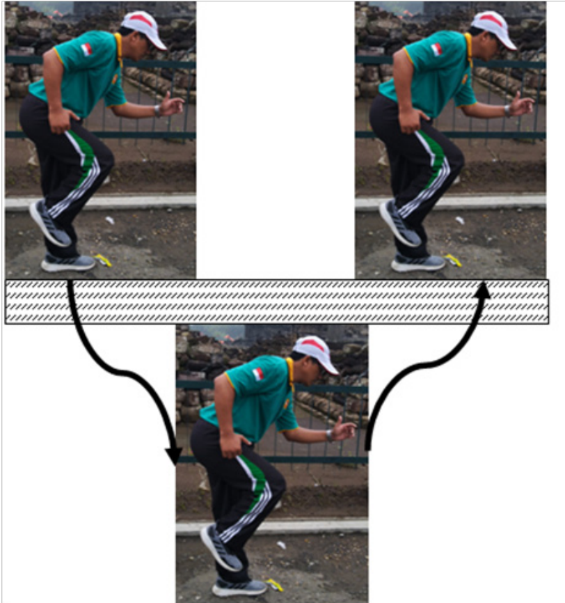
Gambar 2.3 Hop ringan mundur, maju, dan menyamping
